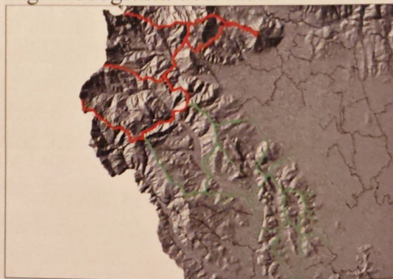
Fig. 4 Orografia dell'area
